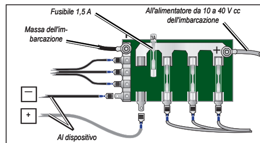
Esempio di blocco fusibili
